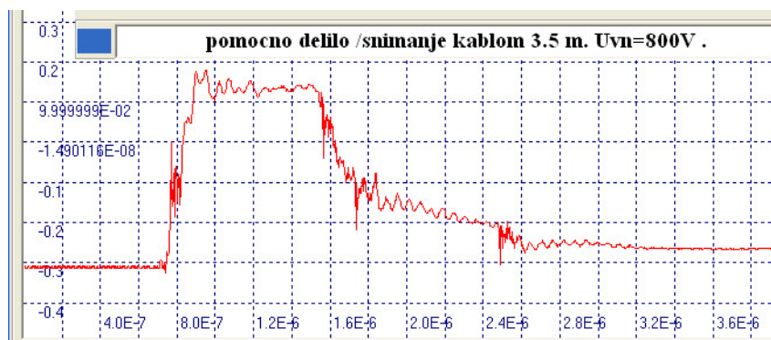
Slika M.28: Odziv na kraju niskonaponskog kabla dužine 3.5 m
