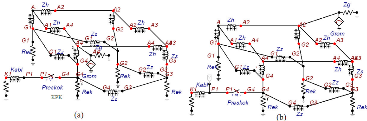
Slika F.6: Ekranski prikaz zamenske šeme kada je udar iznad KPK (a) i na supotnoj strani objekta (b)
