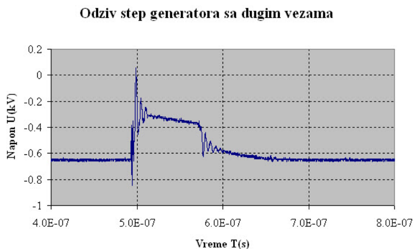
Slika M.4: Snimak oblika koji daje step generator sa dugačkim vezama d_z i d_v
