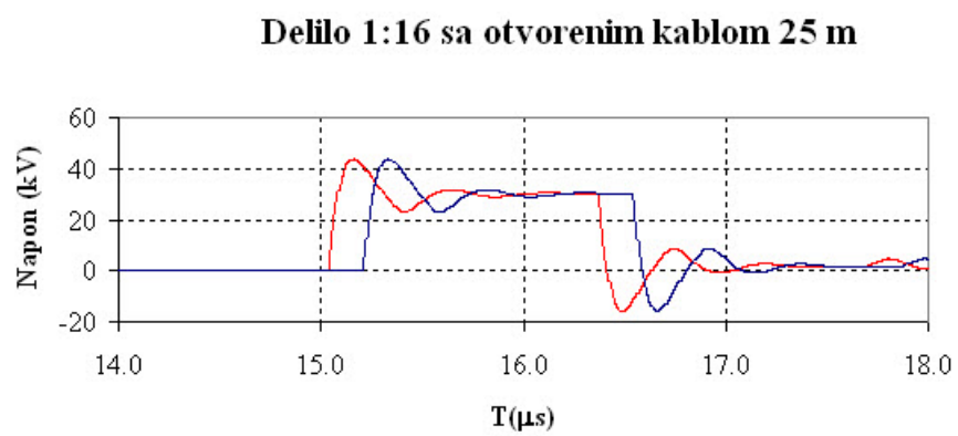
Slika M.25: Talasni oblik napona u tački A16 i na kraju kabla u tački N2 za dužinu kabla 25 m
