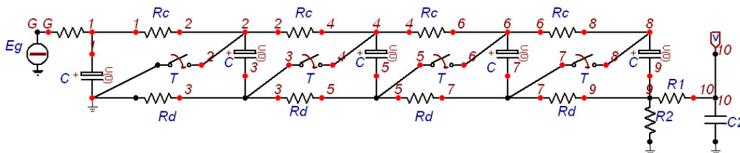
Slika L.3: Ekvivalentna šema 5. stepenog naponskog udarnog generatora
