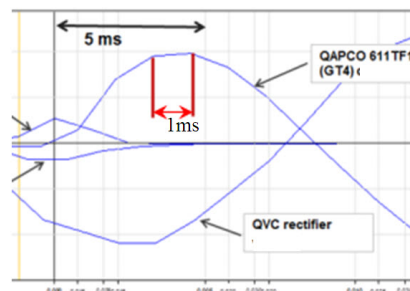
Slika G.7: Procena koraka uzorkovanja merno-akvizicionih sistema relejne zaštite
