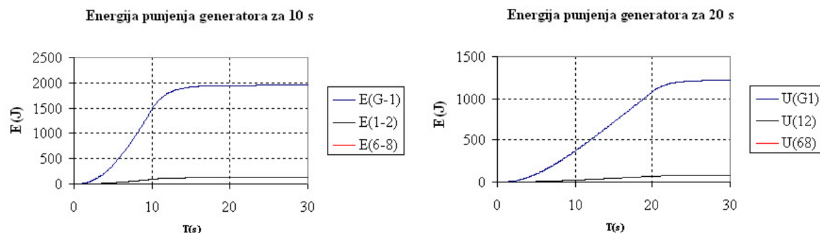
Slika L.9: Energija oslobođena na zaštnomi otporniku, otporniku za punjenje prvog stepena i petog stepena generatora, za 2 različite brzine podizanja napona punjenja
