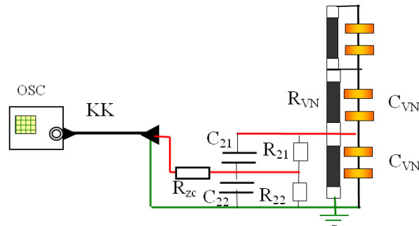
Slika M.26: Delilo napona sa dodatnim delilom u NN grani
