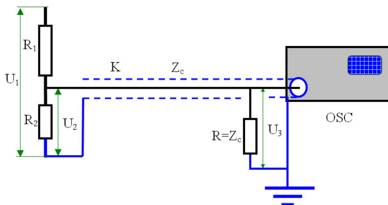
Slika M.1: Merenje udarnog napona pomoću delila i osciloscopa priključenog preko koaksijalnog kabla
