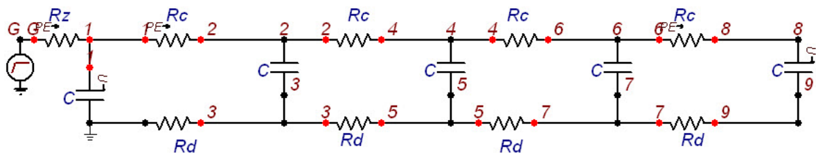
Slika L.6: Zamenska šema udarnog generatora samo sa otpornicima za ograničavanje struje
