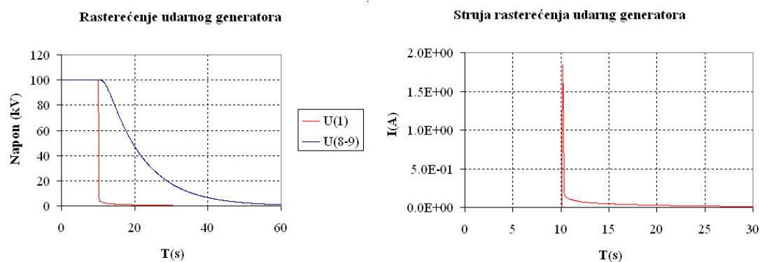
Slika L.14: Talasni oblici napona prilikom uključenja zemljospojnika kada je otpornik za rasterećenje 30 \text{ k}\Omega
