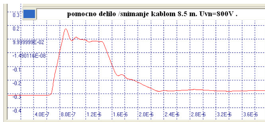
Slika M.32: Odziv na kraju niskonaponskog kabla dužine 8.5 m posle numeričkog filtriranja
