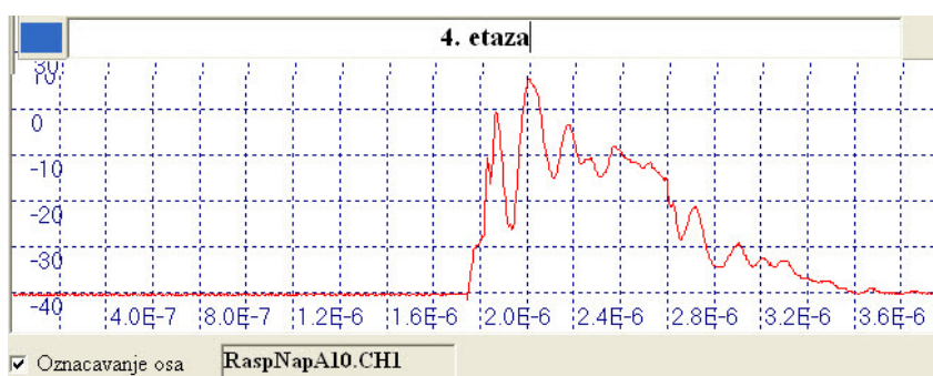
Slika M.13: Odziv na 4. etaži delila
