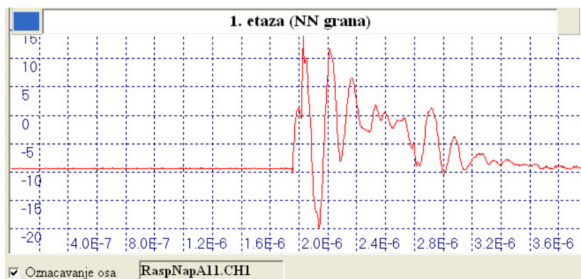
Slika M.14: Odziv na NN grani delila delila
