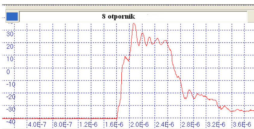
Slika M.12: Odziv na 8. etaži delila
