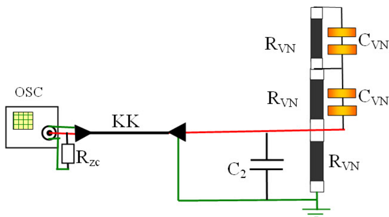
Slika M.16: Veza sa osciloskopom preko koaksijalnog kabla koji je završen prilagodnim otpornikom prema zemlji
