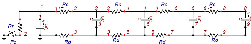
Slika L.11: Šema za modelovanje rasterećenja udarnog generatora u EMTP-atp
