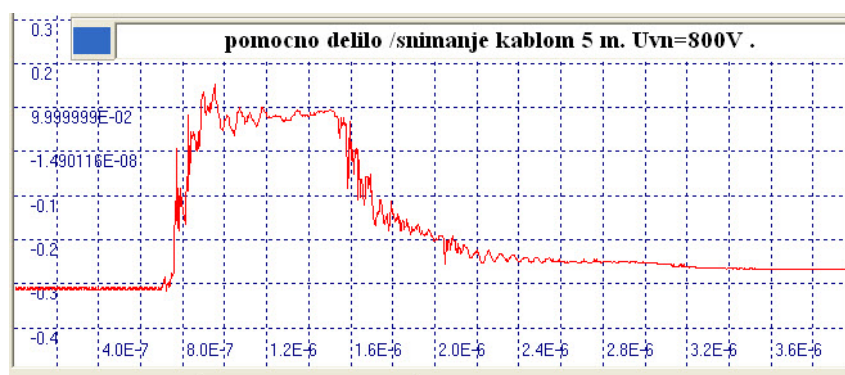
Slika M.29: Odziv na kraju niskonaponskog kabla dužine 5 m
