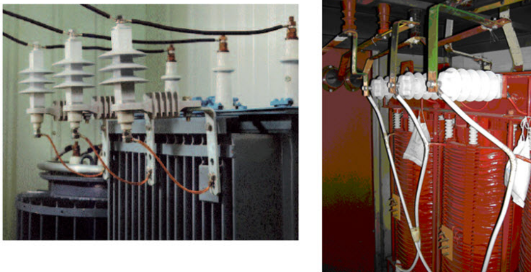
Slika B.11: 1 Slike uljnog i suvog transformatora sa postavljenim odvodnicima prenapona sa silikonskim kućištima direktno na konstrukciji
