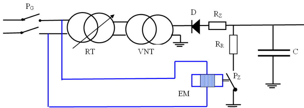
Slika L.10: Šema napajanja generatora i upravljanje zemljospojnikom za rasterećenje generatora
