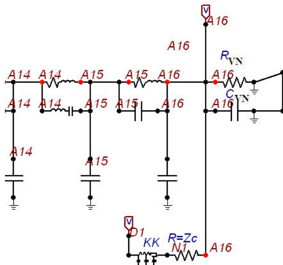
Slika M.22: Zamenska šema donjeg dela delila sa niskonaponskom granom jednakoj visokonaponskoj
