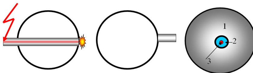
Slika L.2: Troelektrodno iskrište sa internim okidanjem
