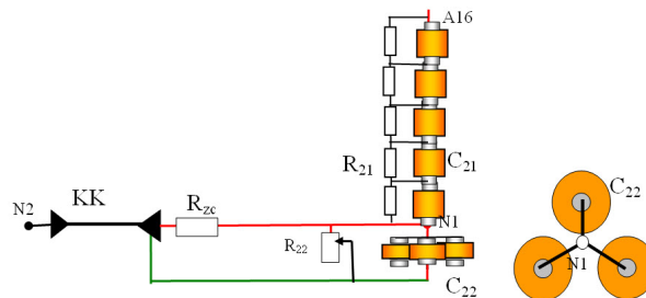
Slika M.27: Izvođenje samo dodatnog delila na niskonaponskoj grani
